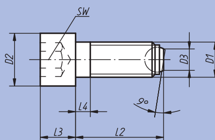
Forme B bille avec plat
