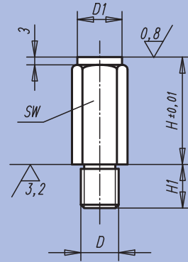
Forme B Surface plane traitée et rectifiée
