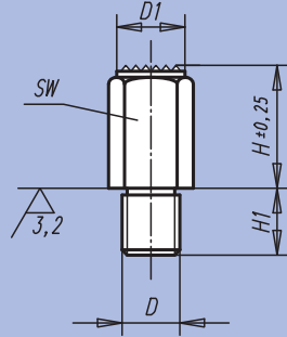
Forme D Surface à picots, trempée
