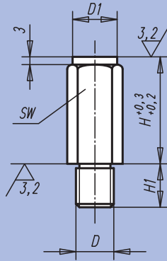
Forme A Surface plane usinée, traîtée
