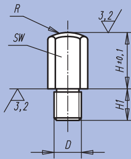
Forme C Surface bombée, traitée
